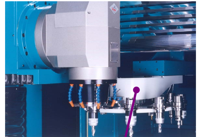
Magazzino Utensili a Ruota Wheel Type Tools Magazine
