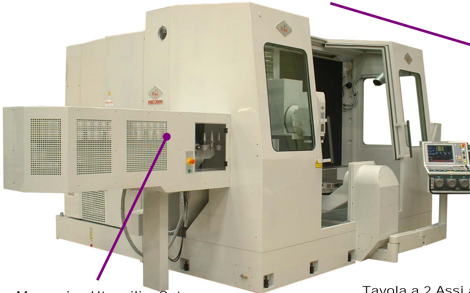
Magazzino Utensili a Catena Chain Type Tools Magazine
